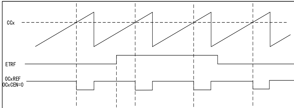
图 58 OCxREF 时序图
