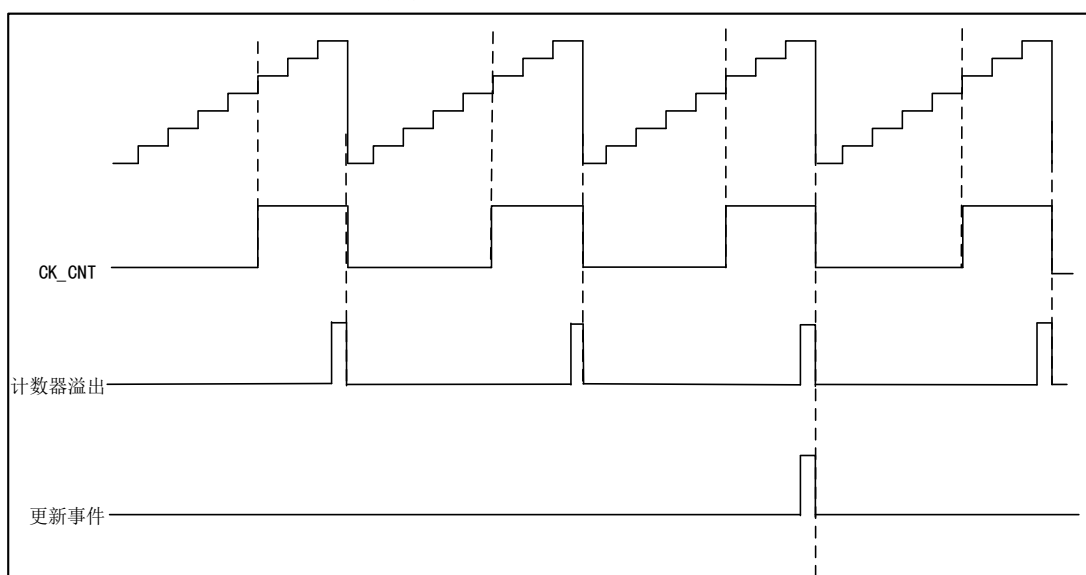
图 67 向上计数模式下，设置 REPCNT=2 的时序图
