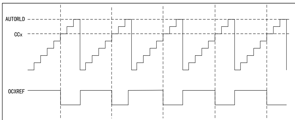
图 27 PWM1 向上计数模式的时序图
