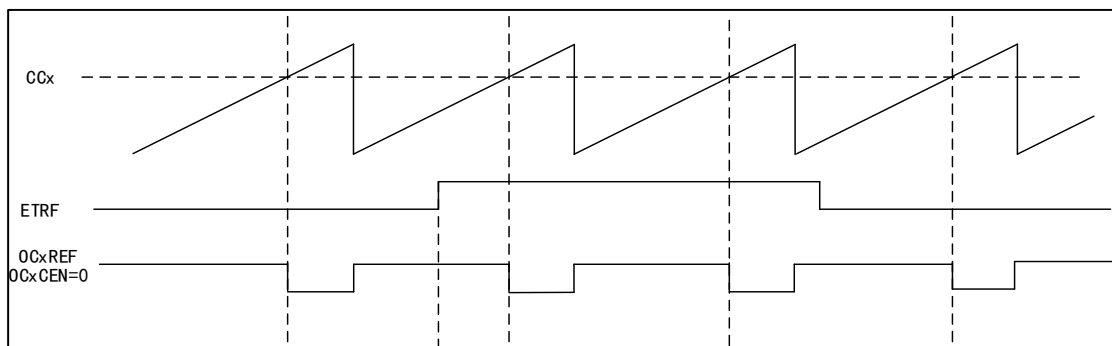
图 41 OCxREF 时序图
