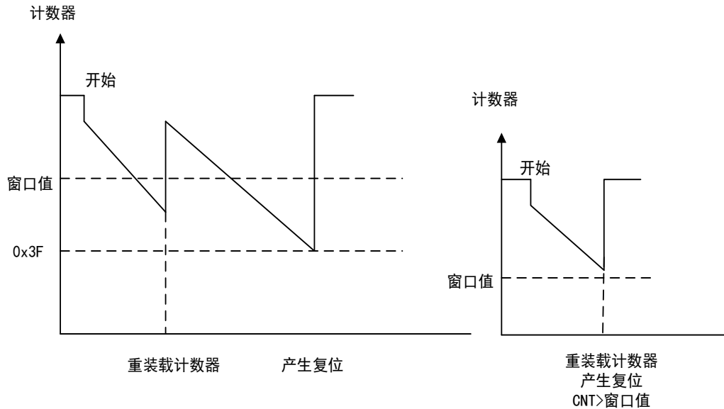
图 81 窗口看门狗时序图
