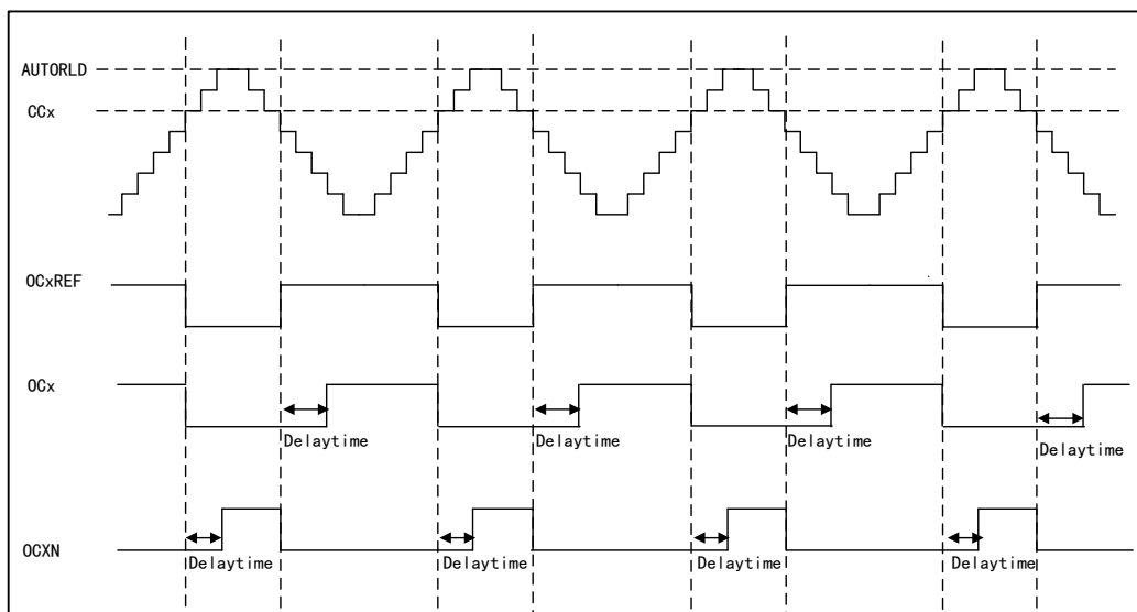
图 74 带死区插入的互补输出
