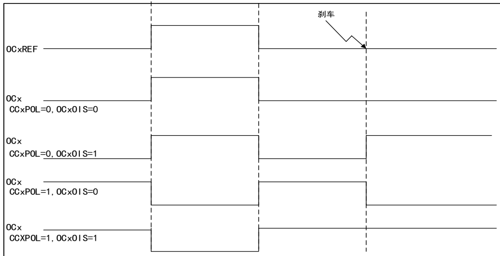
图 73 发生刹车事件的时序图
