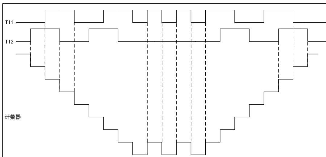
图 39 TI1FP1 反相的编码器接口模式实例
