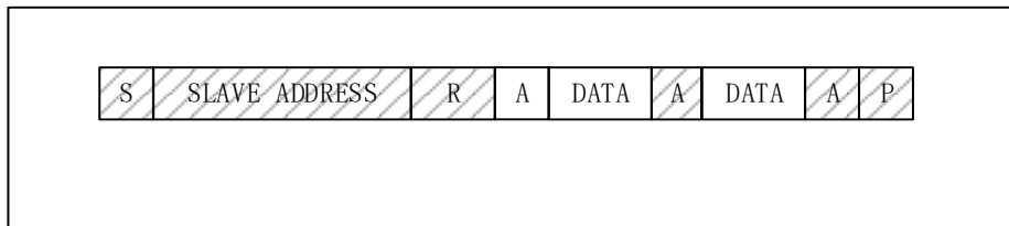
图 94 主机由从机读取数据
