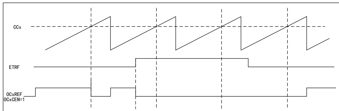
图 42 OCxREF 时序图
