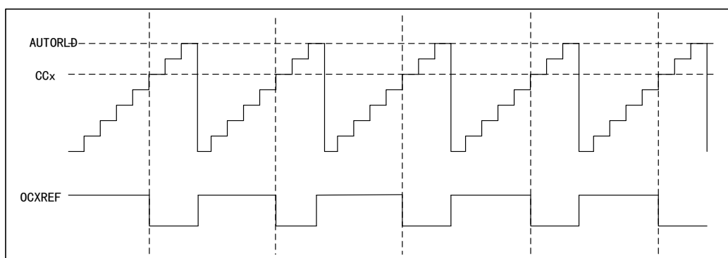
图 62 PWM1 向上计数模式的时序图
