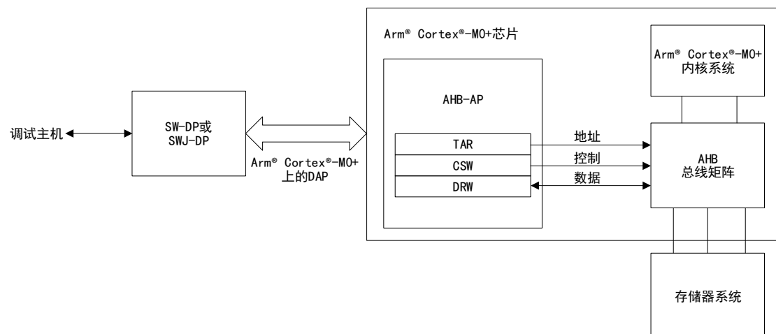
图 15 APM32E0xx 级别和 Arm® Cortex®-M0+级别的调试框图
