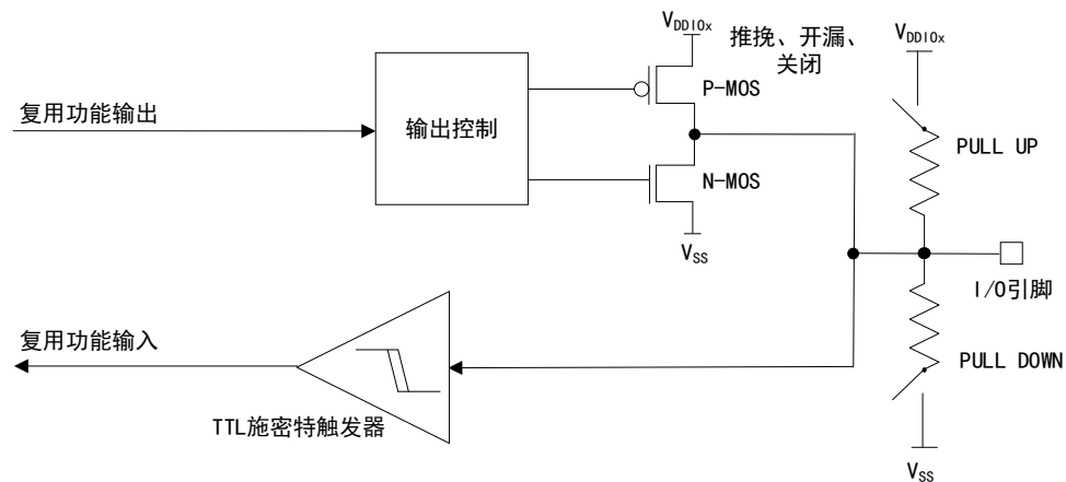
图 21 复用模式下的 I/O 结构
