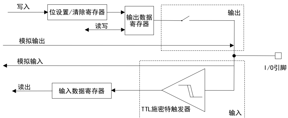
图 20 模拟功能 I/O 结构
