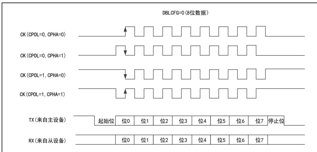
图 86 USART 同步传输时序图 (DBLCFG=0)
