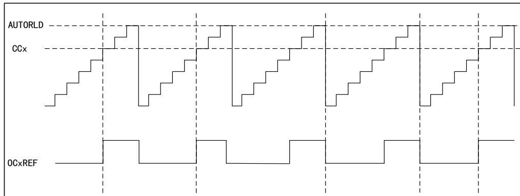
图 63 PWM2 向上计数模式的时序图
