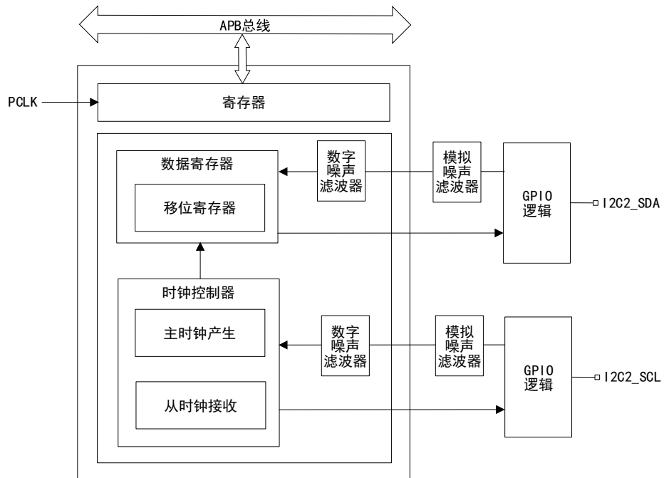
图 91 I2C2 功能结构图
