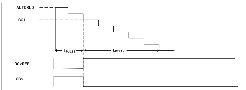
图 54 单脉冲模式下的时序图
