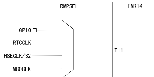
图 5 TMR14 间接测量时钟频率电路图
