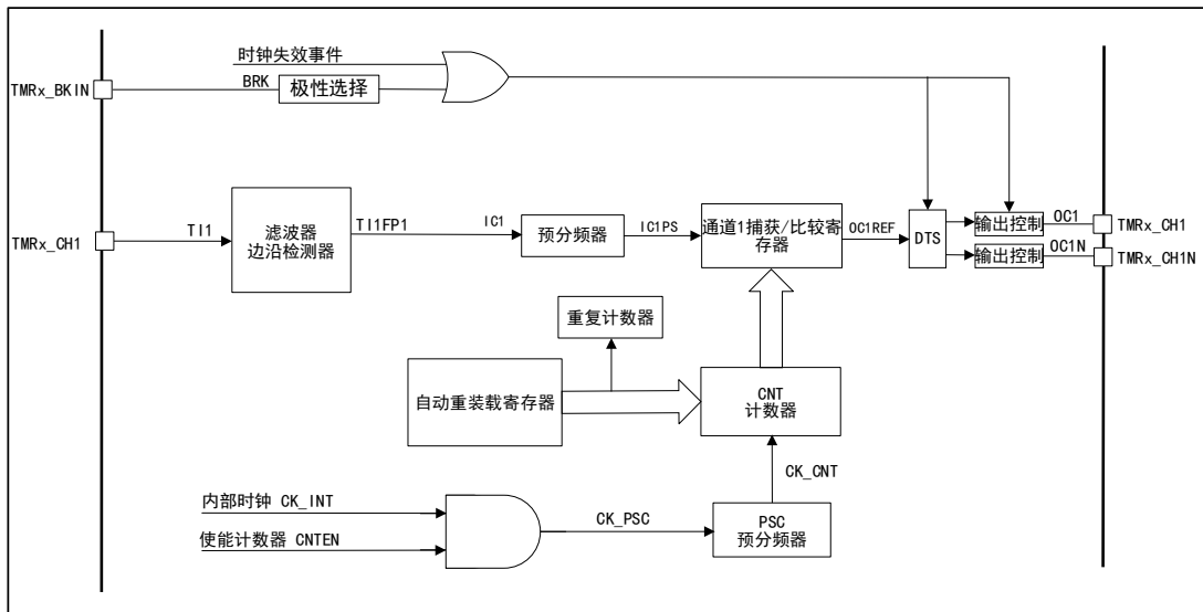
图 65 通用定时器 TMR16/17 结构框图
