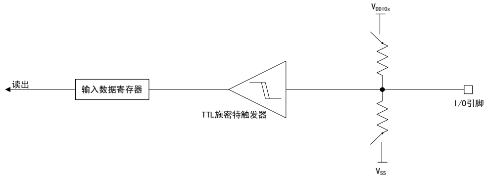
图 17 输入模式 I/O 结构
