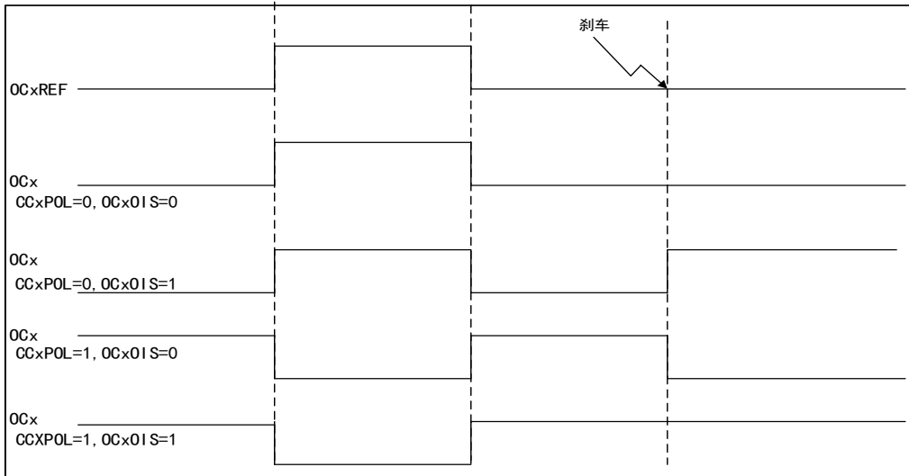
图 36 发生刹车事件的时序图
