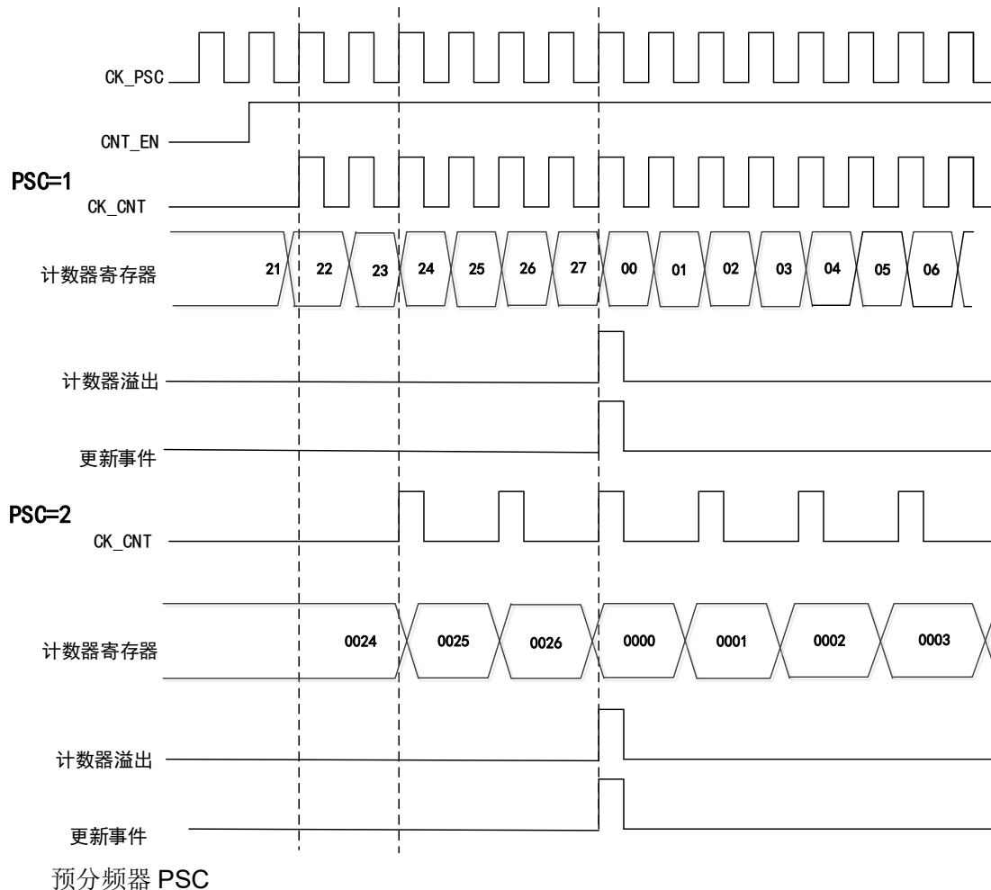
图 61 向上计数模式下，分频因子为 1 或 2 的时序图
