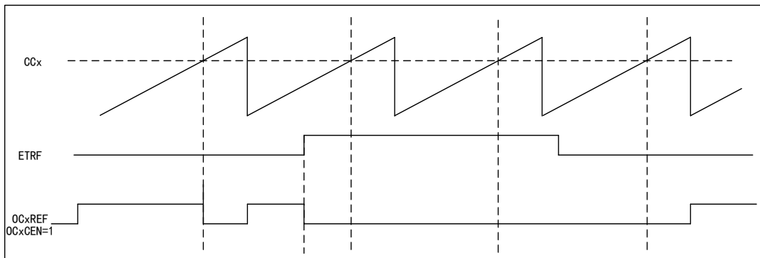
图 59 OCxREF 时序图
