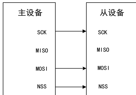
图 98 单工模式连接（主机只发送，从机接收）
