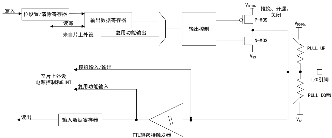
图 16 GPIO 结构框图
