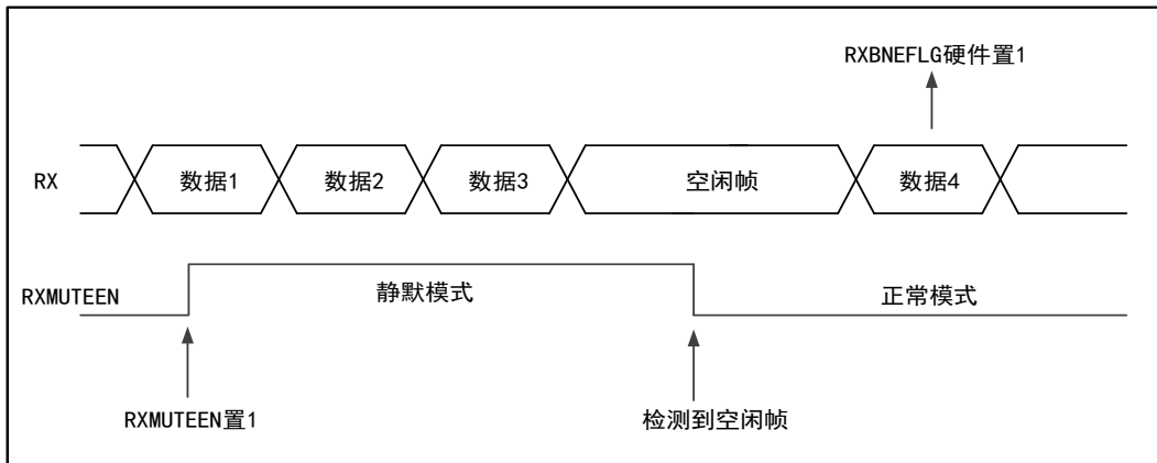
图 83 空闲总线退出静默模式
