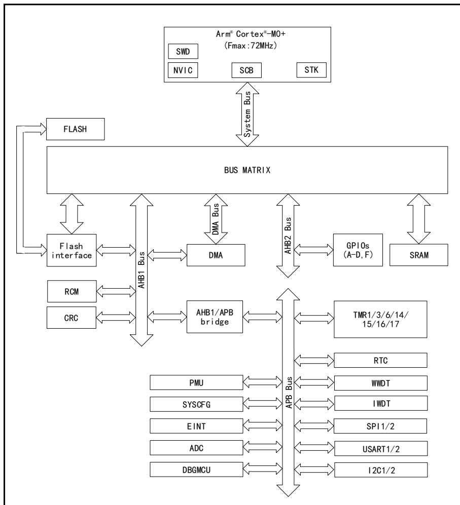
图 1 APM32E030x8 系统架构框图
