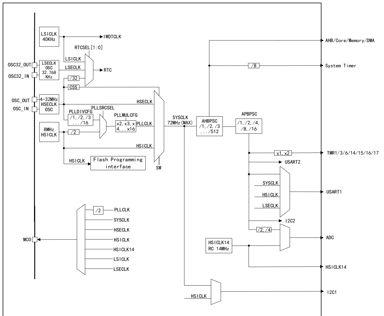
图 4 APM32E030x8 时钟树
