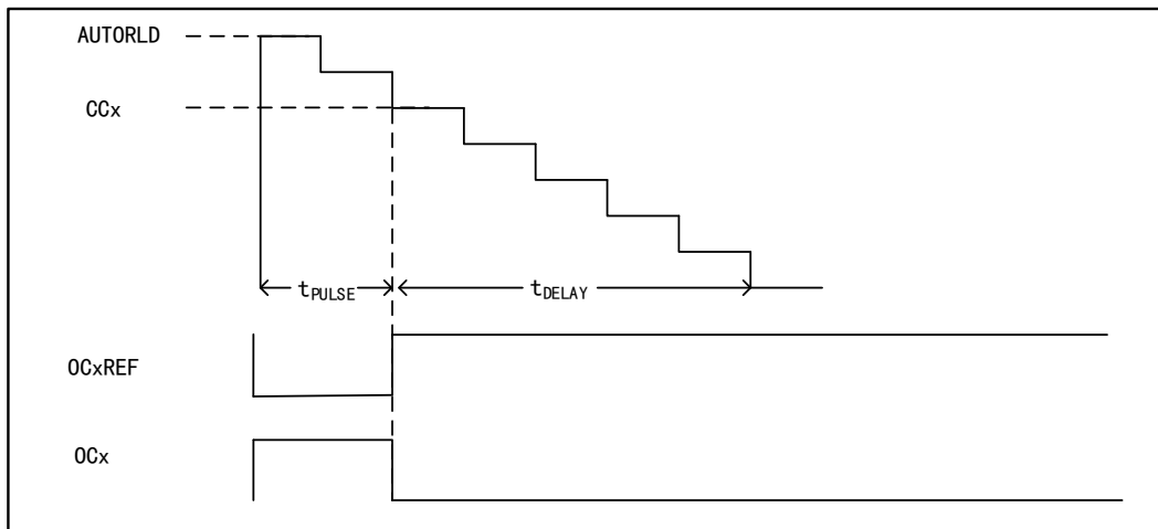
图 34 单脉冲模式下的时序图
