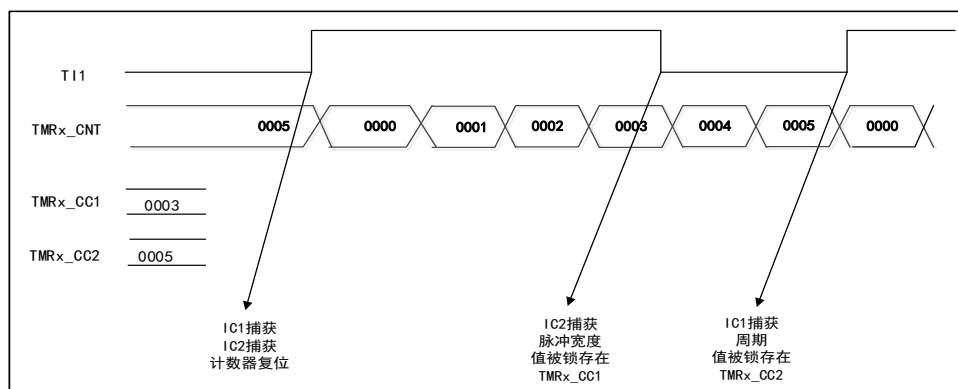
图 53 PWM 输入模式时序图
