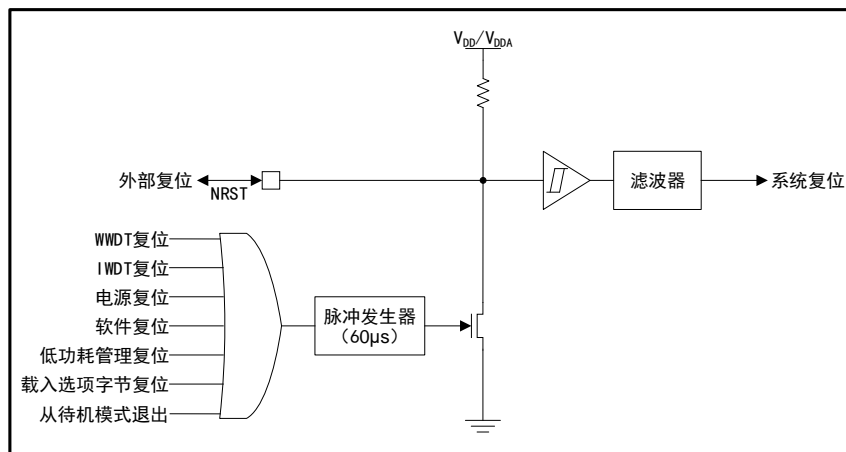
图 2 “系统复位” 复位电路
