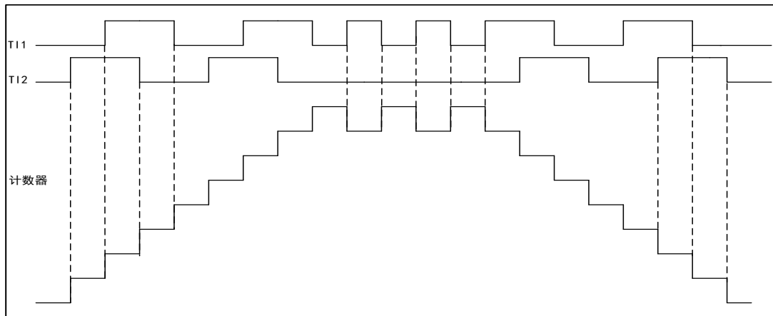
图 55 编码器模式下的计数器操作实例
