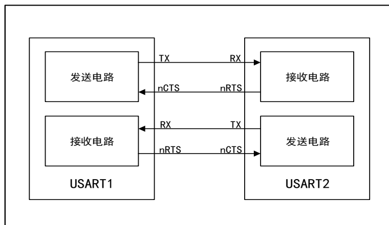
图 88 两个 USART 之间的硬件流控制
