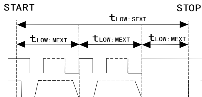
图 95 t_{\text{LOW:SEXT}} 与 t_{\text{LOW:MEXT}} 时间
