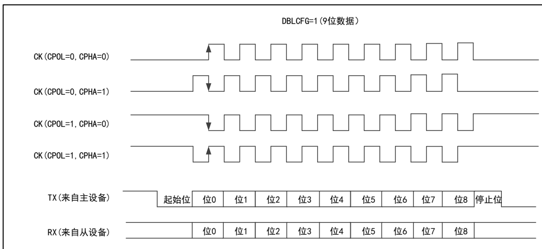
图 87 USART 同步传输时序图 (DBLCFG=1)
