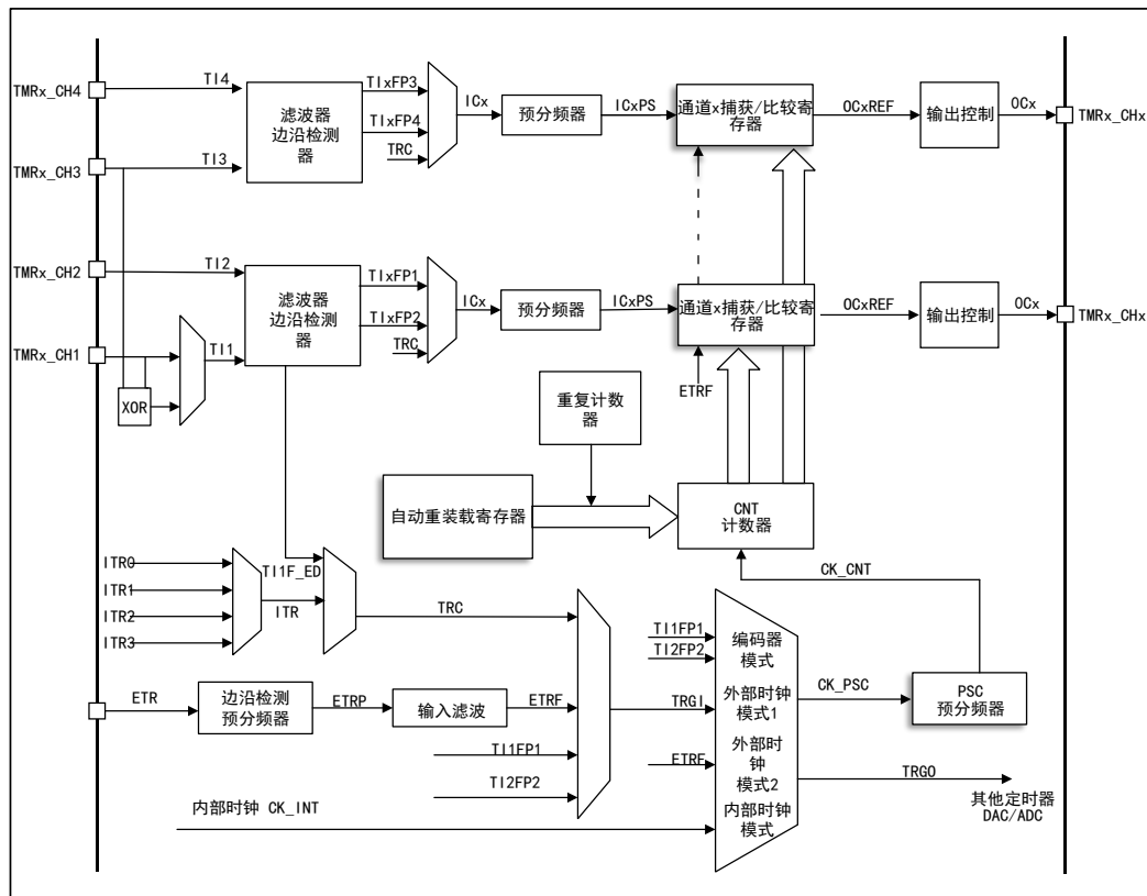
图 43 通用定时器结构框图
