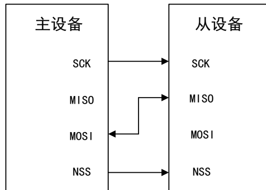
图 99 半双工模式连接
