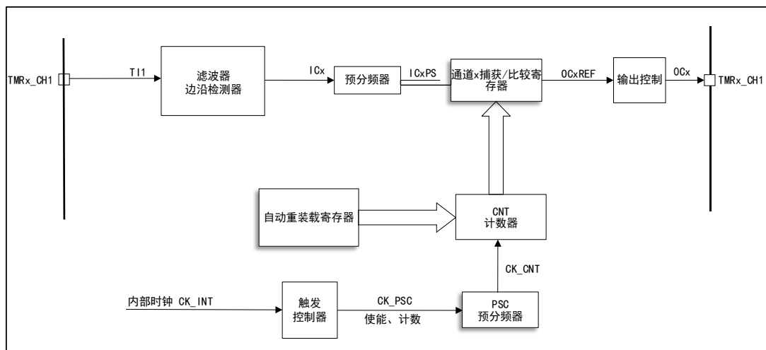
图 60 通用定时器 TMR14 结构框图
