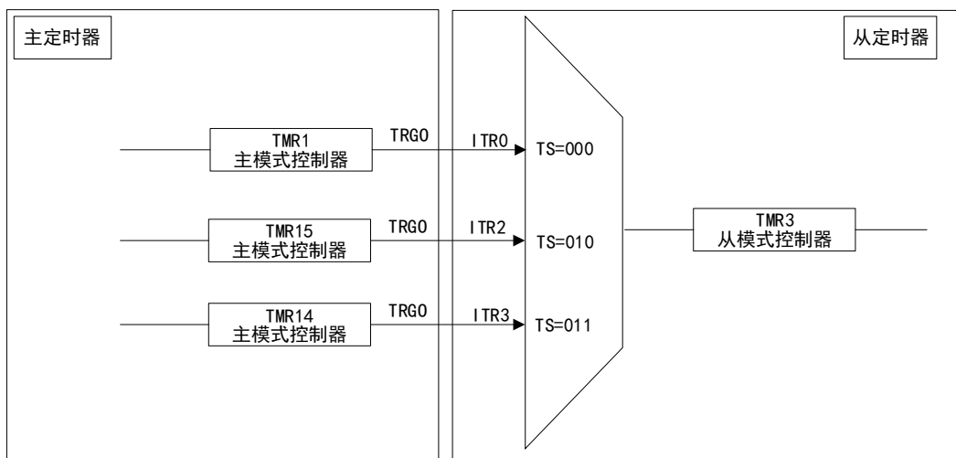
图 57 TMR3 主/从模式的例子
