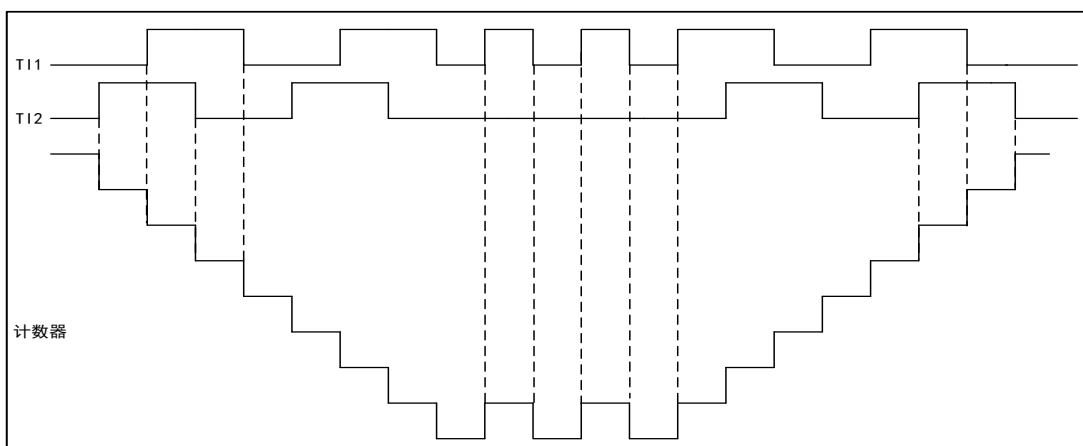
图 56 T11FP1 反相的编码器接口模式实例
