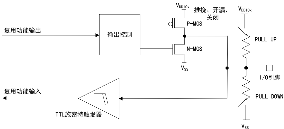
图 19 复用模式 I/O 结构
