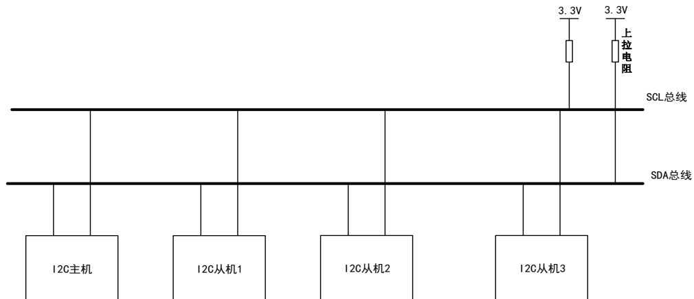
图 92 常见 I2C 通信连接图
