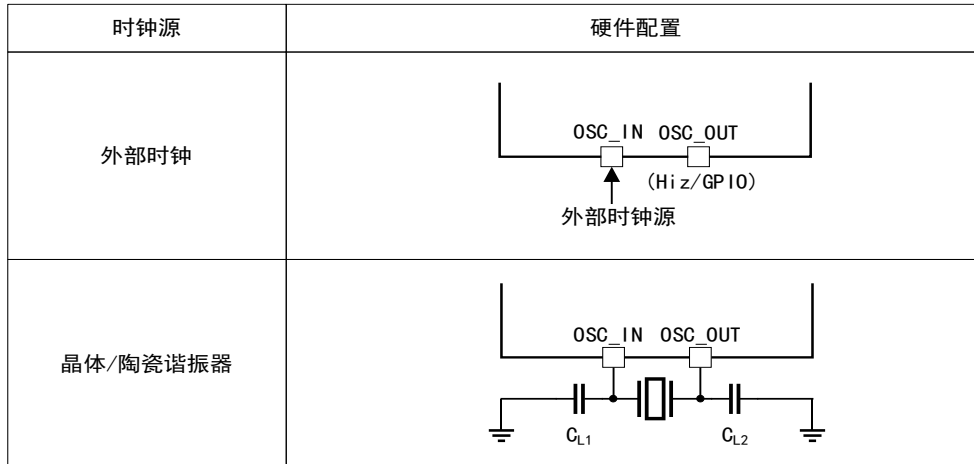
图 3 HSECLK/LSECLK 的时钟源硬件配置
