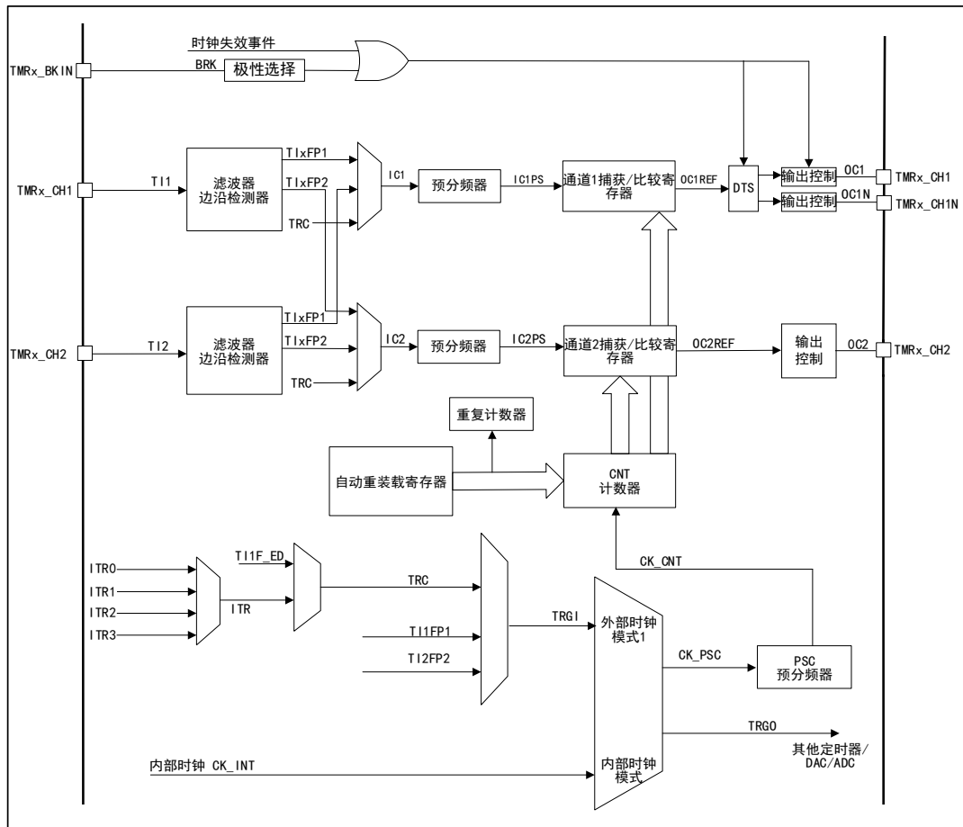
图 64 通用定时器 TMR15 结构框图
