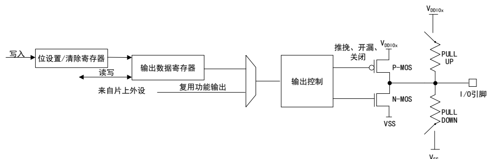
图 18 输出模式 I/O 结构
