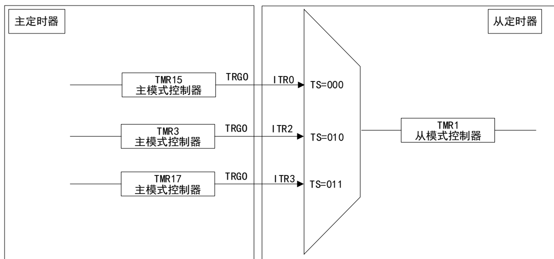
图 40 TMR1 主/从模式的例子
