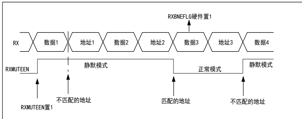
图 84 地址标记退出静默模式
