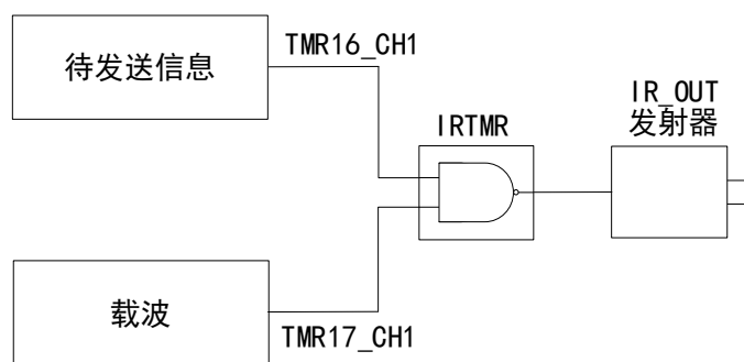
图 78 IRTMR 结构框图
