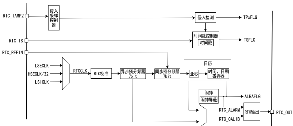
图 82 RTC 结构框图
