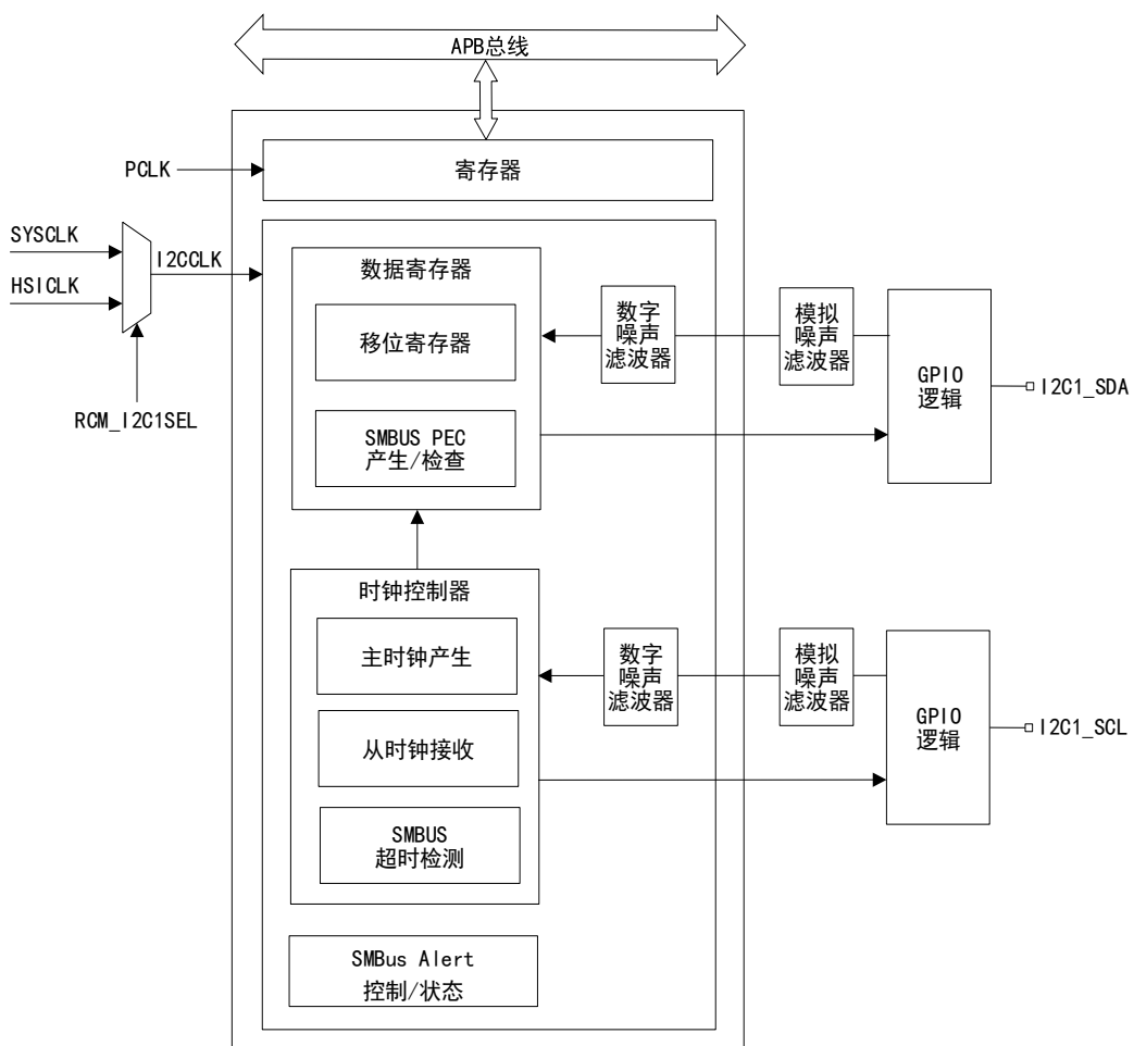
图 90 I2C1 功能结构图
