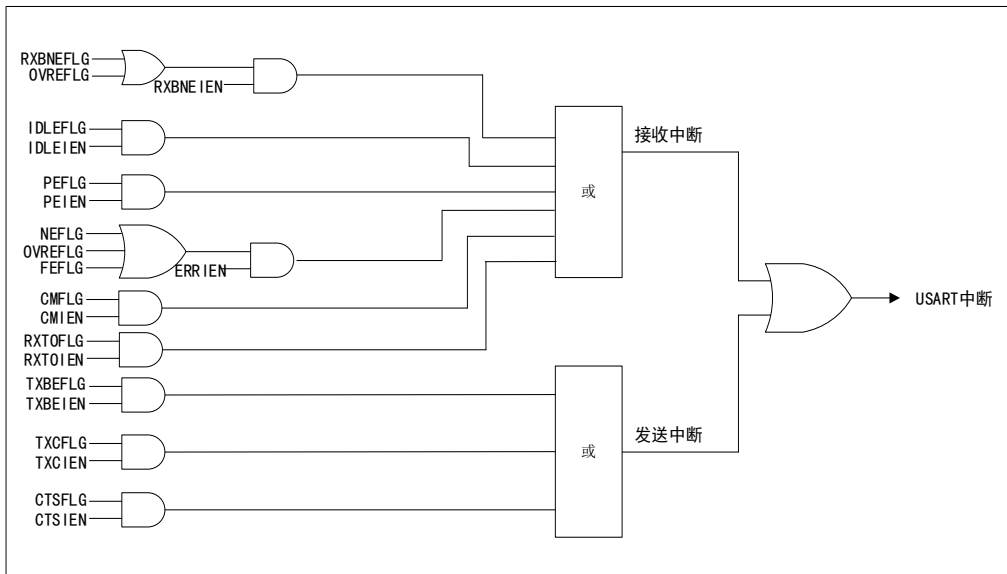
图 89 USART 中断映射
